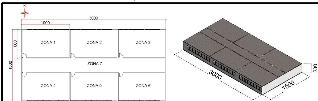
Figura 1 - Planta baixa e modelo
